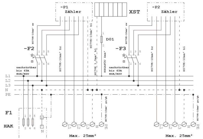
2 Zählerplätze TN-C-S System + TSG Absicherung D01
